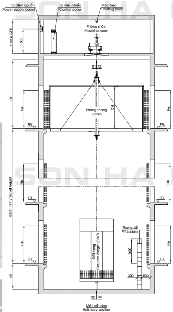
THANG CÓ PHÒNG MÁY / MACHINE ROOM ELEVATOR
