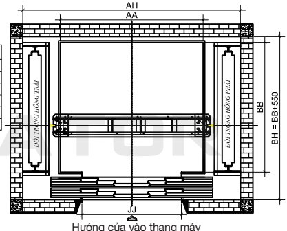
HỒ THANG TẢI HÀNG 1 ĐẾN 5 TẦN ĐỐI TRỌNG NẪM HÔNG CỬA CO-6 CẢNH MỜ TİM
