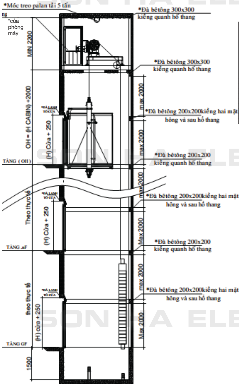
HỒ THANG TẢI HÀNG 1 ĐẾN 5 TẦN ĐỐI TRỌNG NẪM HÔNG CỬA CO-4 CẢNH MỜ TİM
