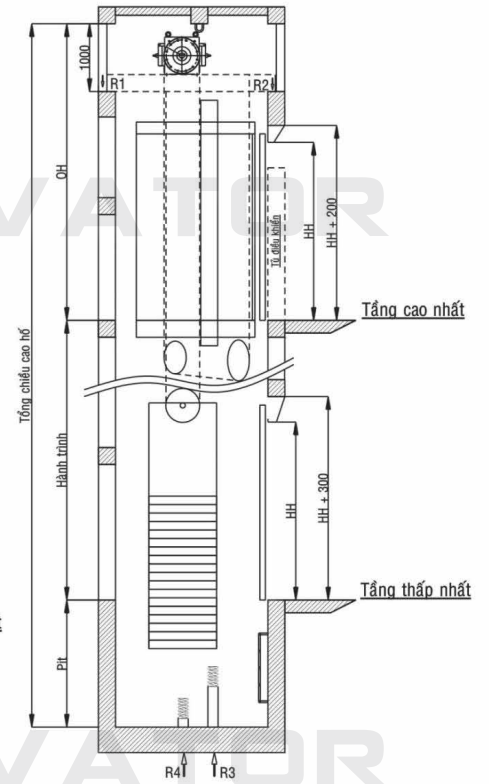
Thang không phòng máy Elevator without engine room
