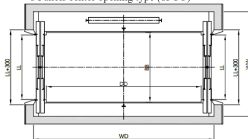
Kiểu cửa 3 cánh đóng mở theo phương đứng (3U) 3 Panels upsliding type (3U)
