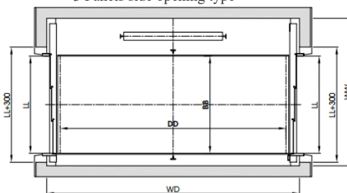
MẶT BẰNG ĐIỂN HÌNH / TYPICAL PLAN
