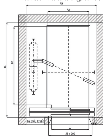
Thang không phòng máy Elevator without engine room
