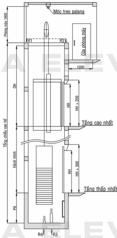
Thang có phòng máy Elevator has engine room
