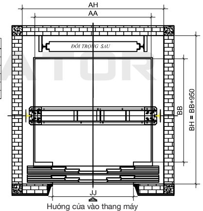
HỒ THANG TẢI HÀNG 1 ĐẾN 5 TẦN ĐỐI TRỌNG NẪM HÔNG CỬA CO-6 CẢNH MỜ TİM
