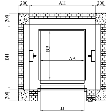
THANG TẢI THỰC PHẨM KHÔNG ĐỐI TRỌNG
