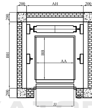
THANG TẢI THỰC PHẨM CÓ ĐỐI TRỌNG
