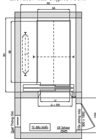
Thang có phòng máy Elevator has engine room
