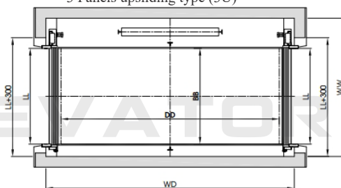
Kiểu cửa 3 cánh đóng mở về 1 phía 3 Panels side opening type
